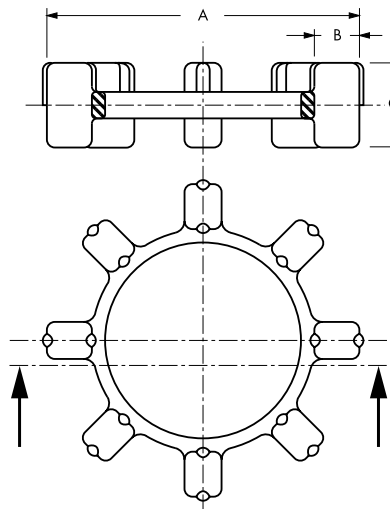
Sizes Tailles 4 - 135 Baugröße
