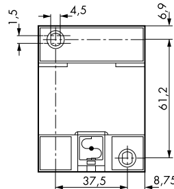
Drehzahlwächter
