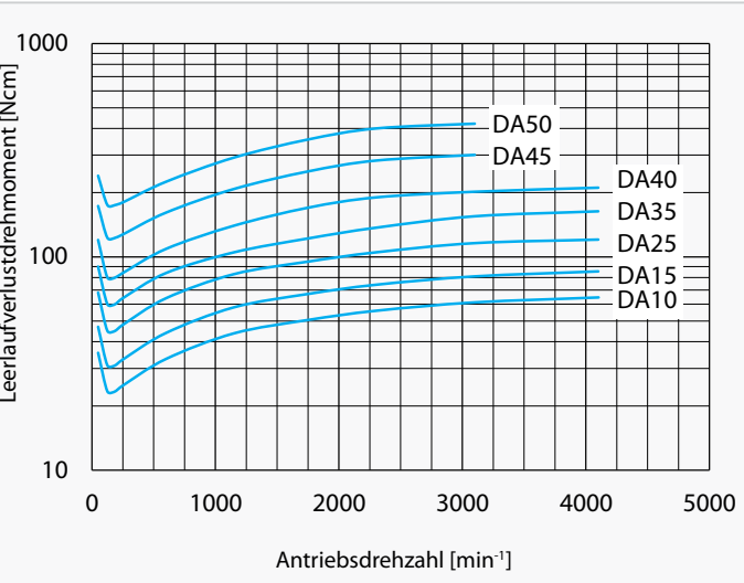
Abb. DA-1 Antriebsseitiges Leerlaufverlustdrehmoment
