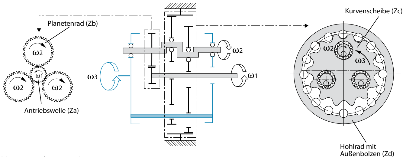
Abb. 5 Zweistufiges Getriebe
