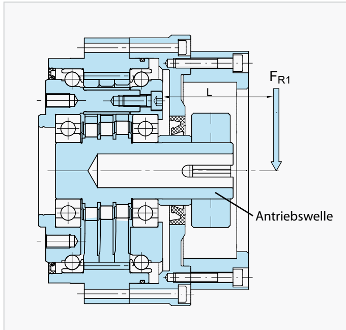
Abb. DA-4 Lastangriff an Antriebswelle
