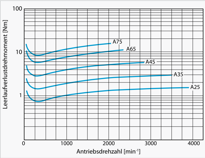
Abb. A-2 Antriebsseitiges Leerlaufverlustdrehmoment (i 29)
