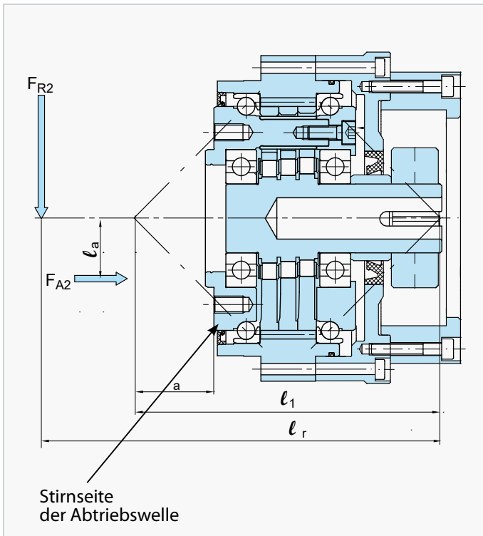
Abb. DA-5 Lastangriff Abtrieb
