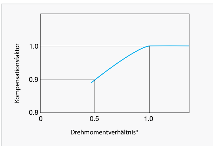
Abb. A-4 Kompensationskurve für Wirkungsgrad
