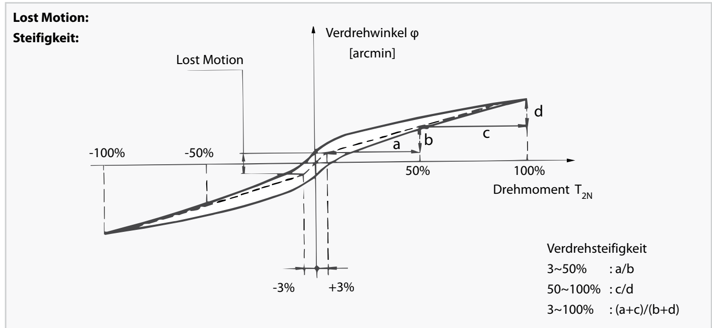
Abb. 7 Hysteresekurve
